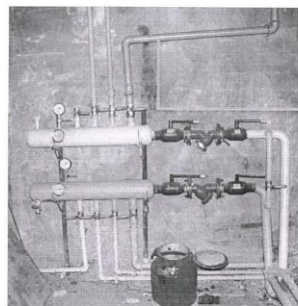
Шинээр хийсэн Ф50мм –ийн халаалтын өгөх шугам
