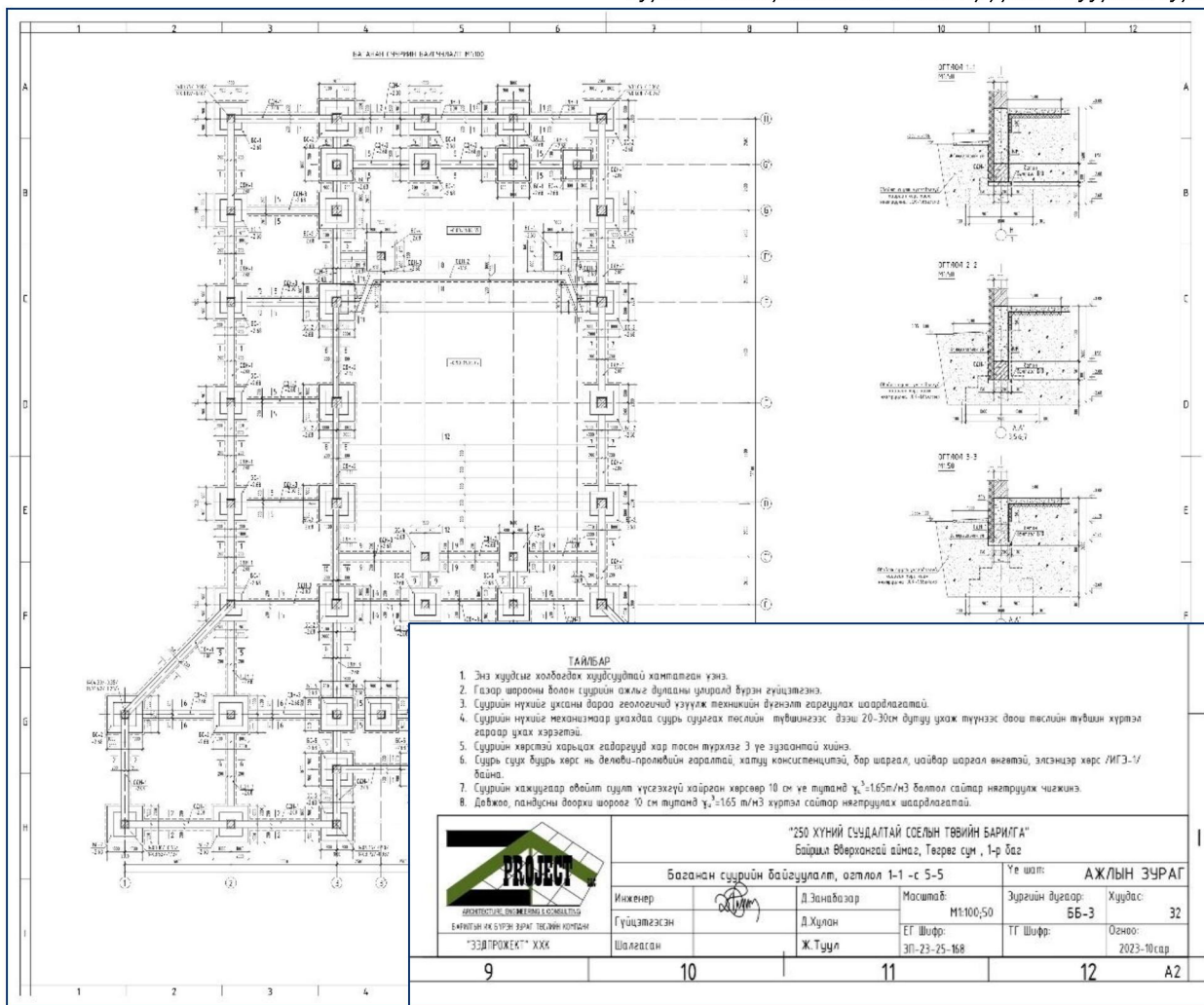
Зураг 2. Зэдпроект ХХК-аас ирүүлсэн суурийн зураг
