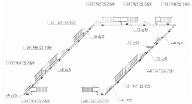
Зураг №4 Тариалан сумын Цаг Уурын өртөөний барилга халаалтын зуух, систем
