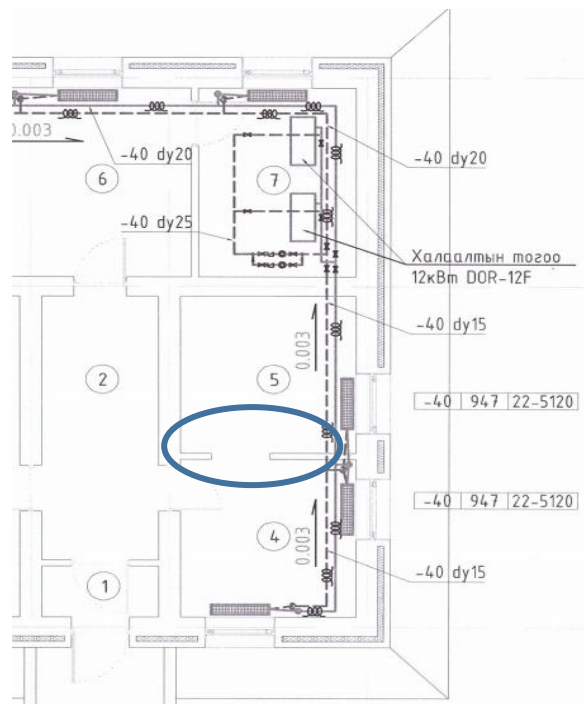
Зураг №2 Шинэ-Идэр сумын Цаг-Уурын өртөөний барилга
