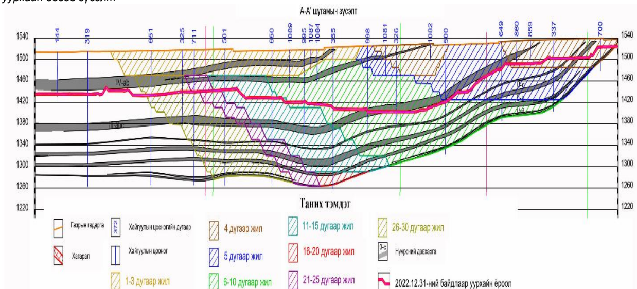
Зураг 2а. Цанхийн зүүн уурхайн анхны ТЭЗҮ-эрх төлөвлөлт 2011 он, 2022 оны 12 дугаар сарын 31-ний өдрийн байдлаарх уурхайн босоо зүсэлт
